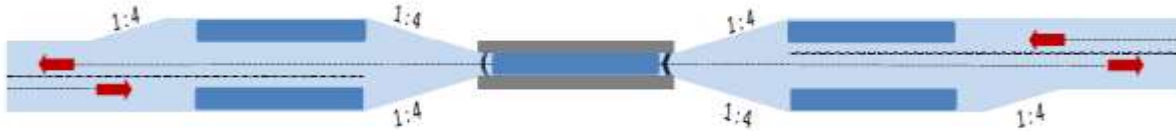
Abb. 2 Verschwenkung der Kanalachse in Vorhäfen einer Einzelschleuse (Prinzip-Skizze)
