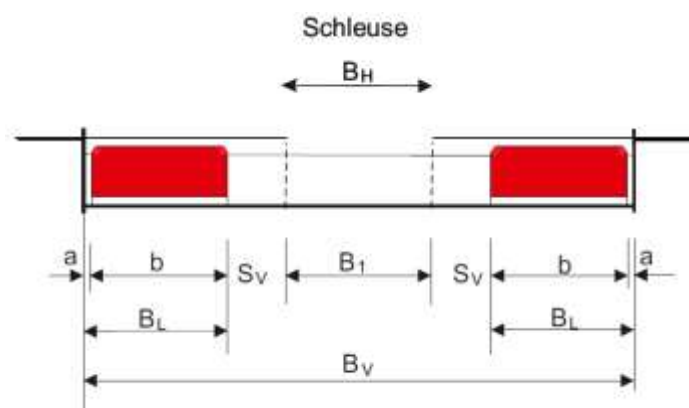
Abb. 3 Querschnitt des Vorhafens einer Einzelschleuse mit beidseitigen Liegeplätzen
